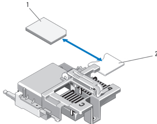
Abbildung 14. Austauschen der vFlash SD-Karte
