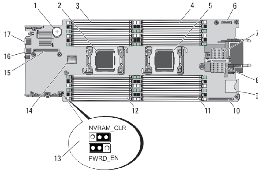
Abbildung 25. Anschlüsse auf der Systemplatine
