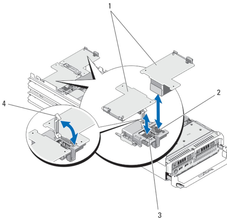
Abbildung 11. Entfernen und Installieren einer PCIe-Zusatzkarte
