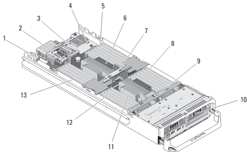
Abbildung 7. Im Inneren des Servermoduls
