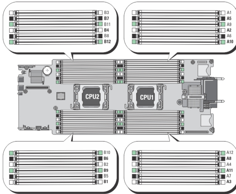
Abbildung 9. Positionen der Speichersocket
