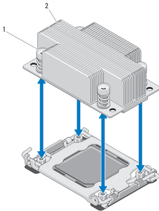
Abbildung 16. Installieren und Entfernen eines Kühlkörpers
