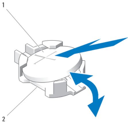
Abbildung 23. NVRAM-Stützbatterie austauschen
