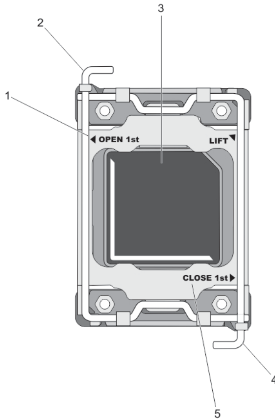
Abbildung 17. Abfolge der Hebel beim Öffnen und Schließen der Prozessorabdeckung
