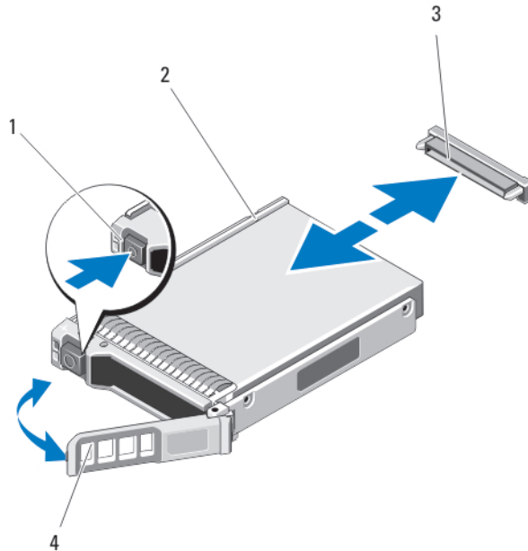
Abbildung 19. Festplatten-/SSD-Laufwerk entfernen und installieren
