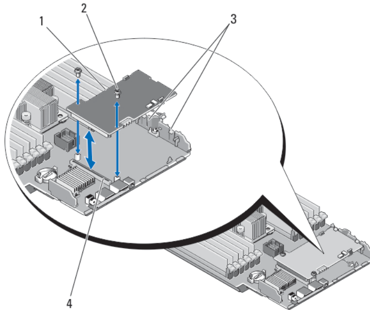
Abbildung 24. Die Speichercontrollerkarte entfernen und installieren
