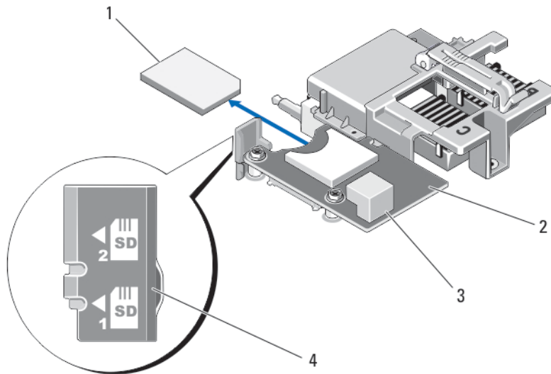
Abbildung 12. Austauschen der SD-Karte
