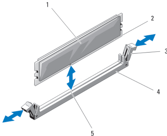
Abbildung 10. Installieren und Entfernen eines Speichermoduls oder einer Speichermodulplatzhalterkarte
