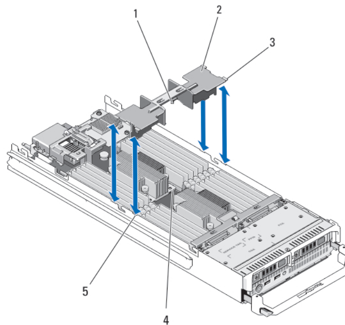
Abbildung 8. Kühlgehäuse installieren und entfernen
