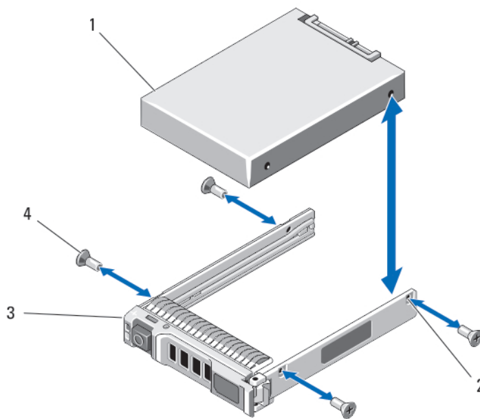
Abbildung 20. Entfernen und Installieren eines Festplatten-/SSD-Laufwerks aus/in einem Festplatten-/SSD-Laufwerksträger
